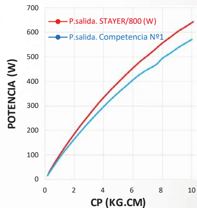
COMPARATIVA TORQUE (Kg.cm) Vs POTENCIA MECÁNICA DE SALIDA (W)
