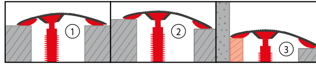
3in1 Profil: (1) Übergangsprofil, (2) Anpassprofil und (3) Abschlussprofil in einem
